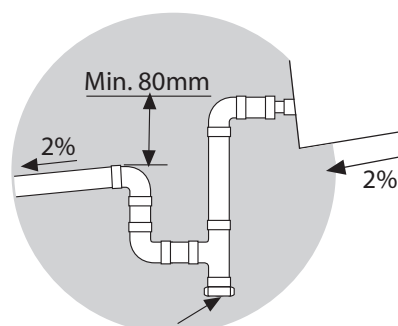
Tappo di ispezione e pulizia
